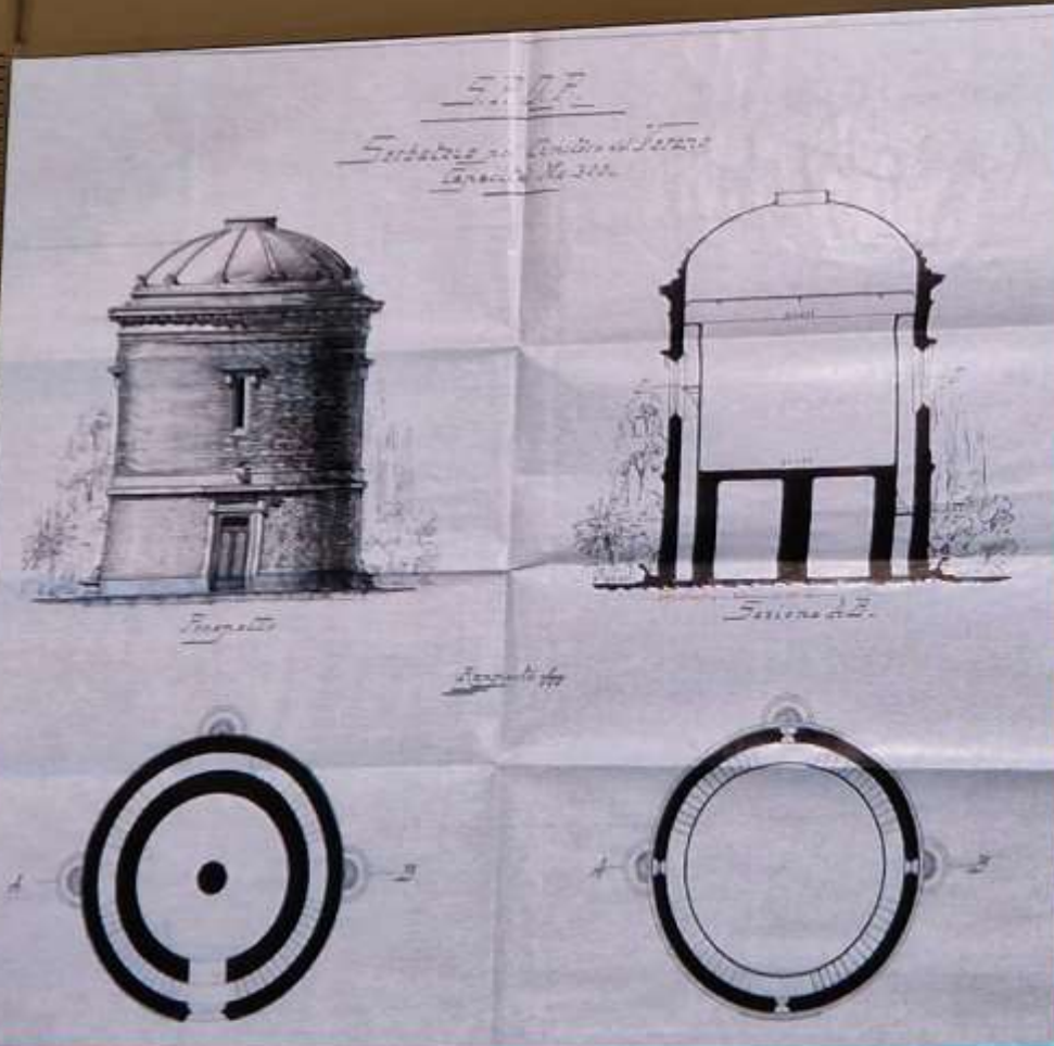
Emilio Saffi, Progetto per il serbatoio idrico del cimitero del Verano, 1906, ASC.
