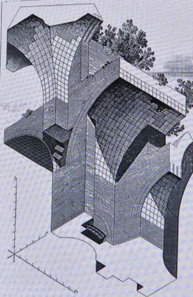
Auguste Choisy, L'Art de bâtir chez les Romains , 1873
